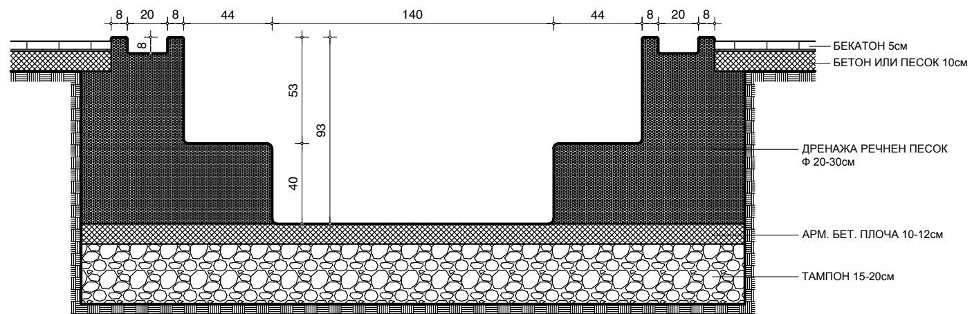
ПРЕСЕК
